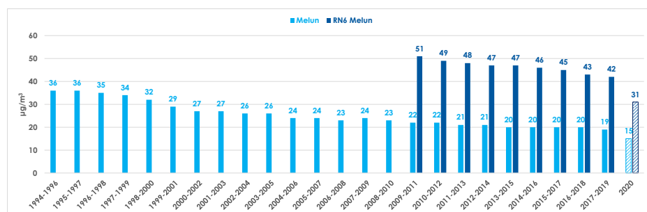
Évolution de la concentration moyenne 3 ans en NO 2 en fond et en trafic dans le territoire de Melun Val de Seine (station de fond Melun et station trafic RN6 Melun)
